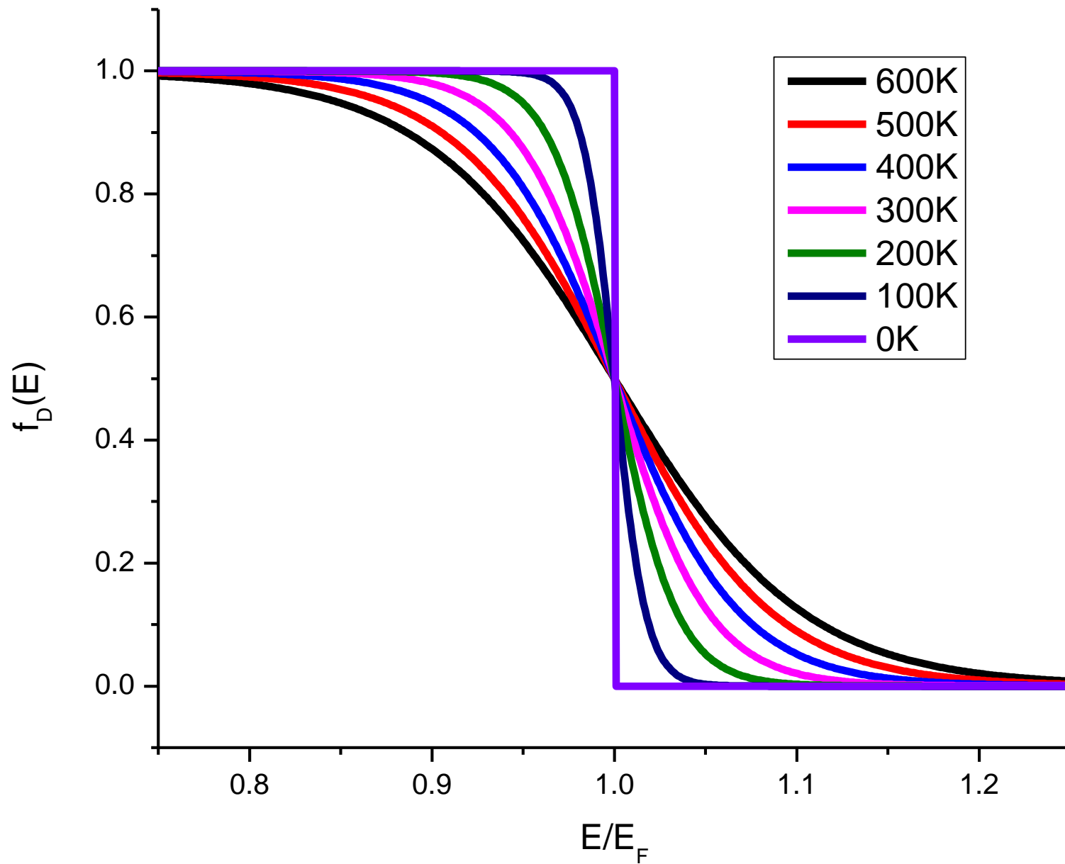
Fermi-Dirac Distribution ( f_D(E) )
