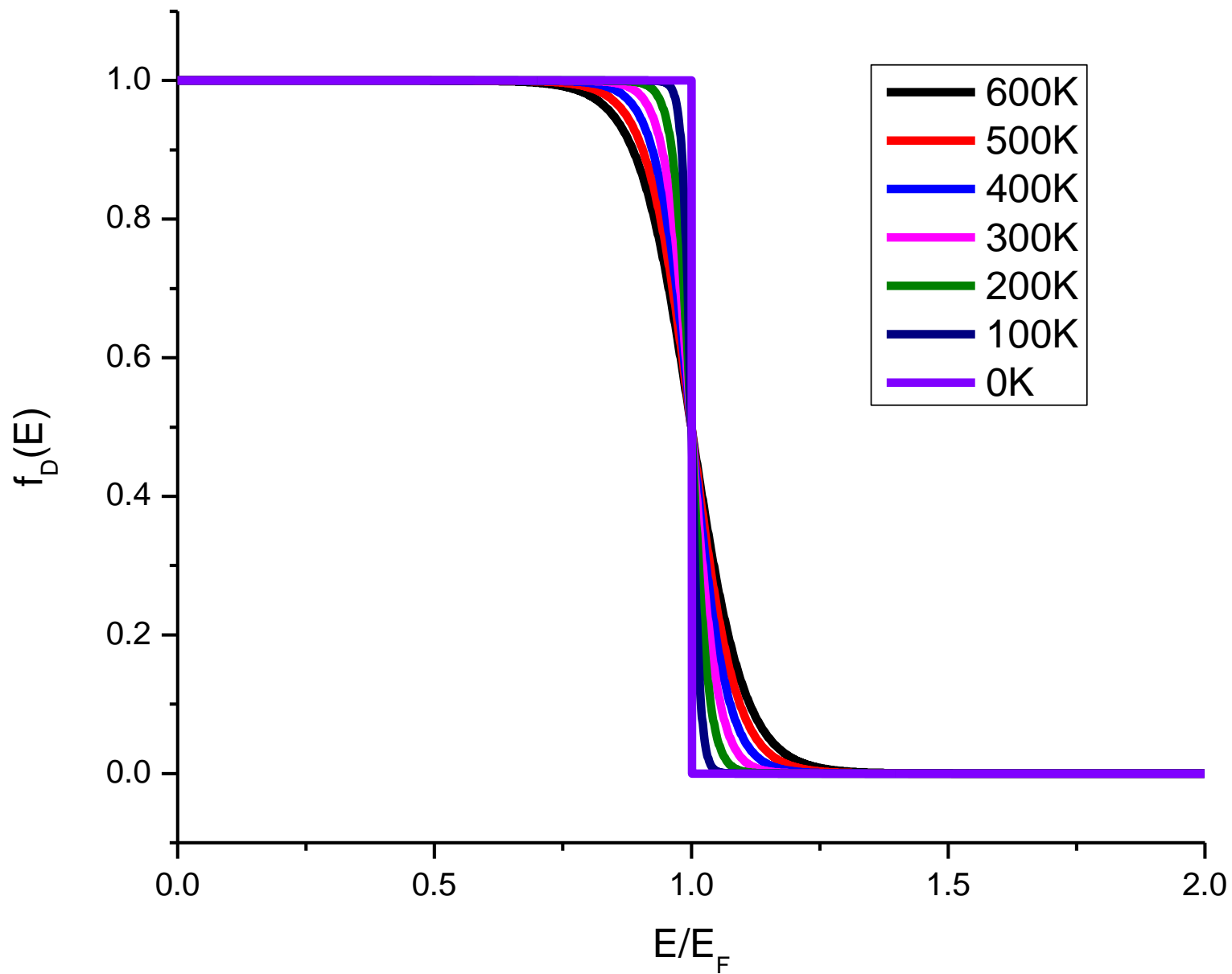
Fermi-Dirac Distribution ( f_D(E) )
